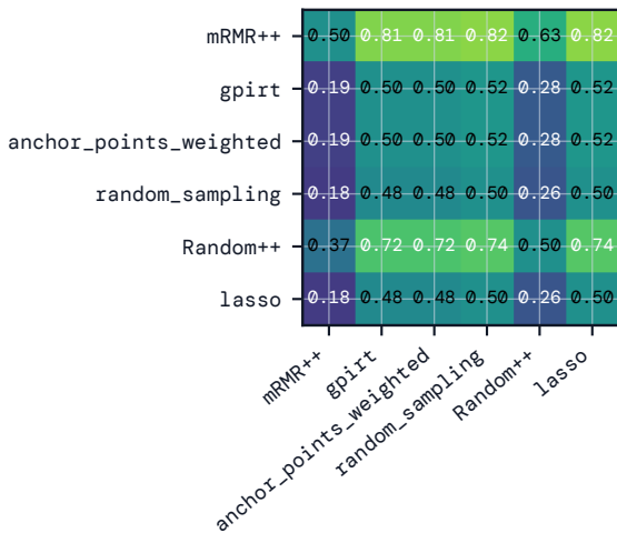
(d) Spearman \rho pairwise
