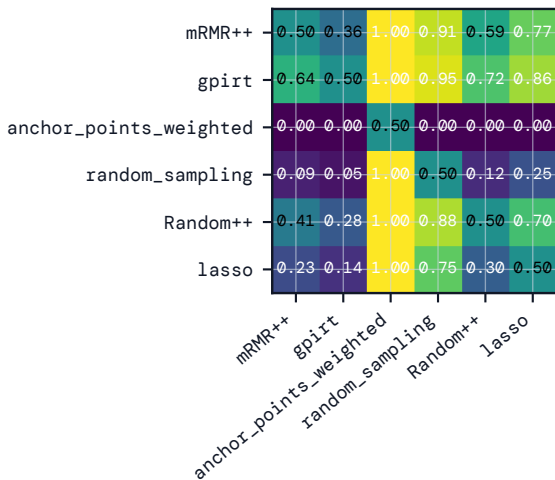
(b) MAE (%) pairwise
